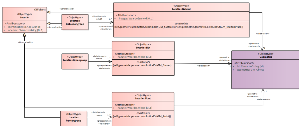
Figuur 4: UML-diagram bij Locatie
