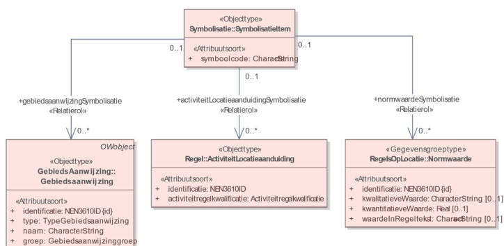
Figuur 11: SymbolisatieItem en de verwijzing naar OW-objecten
