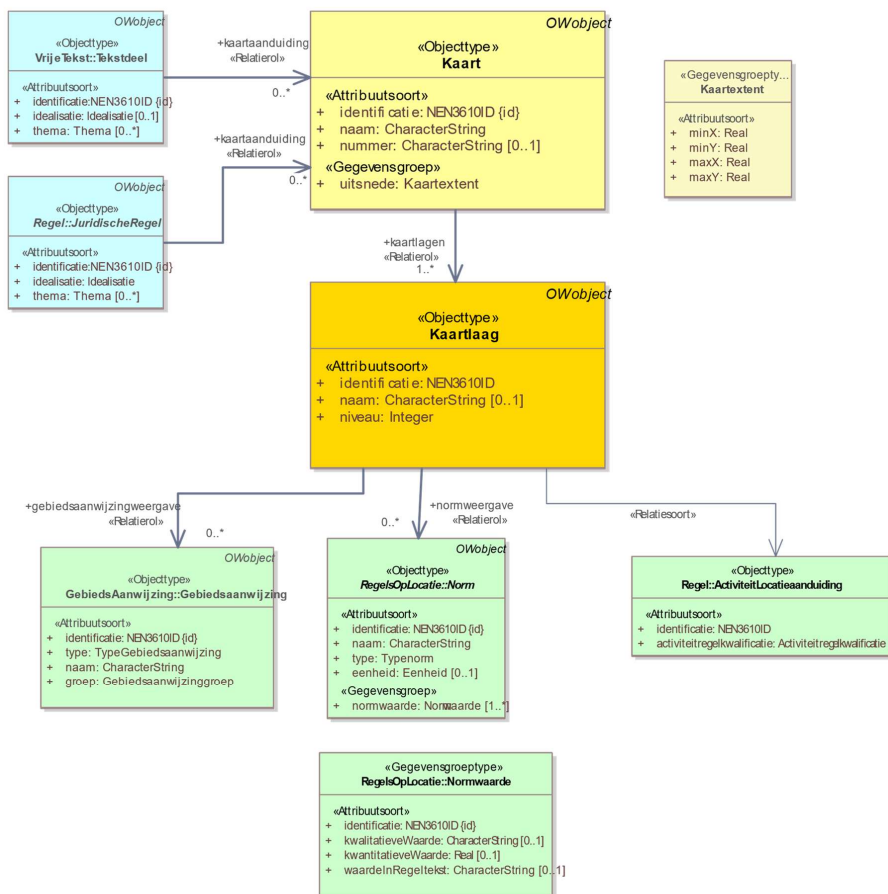
Figuur 16: het informatiemodel van het OW-object Kaart
