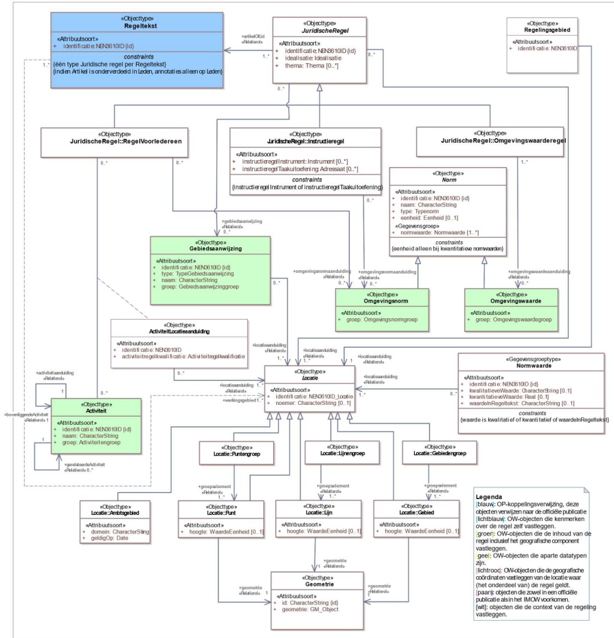
Figuur 8: Het IMOW-diagram in UML.
